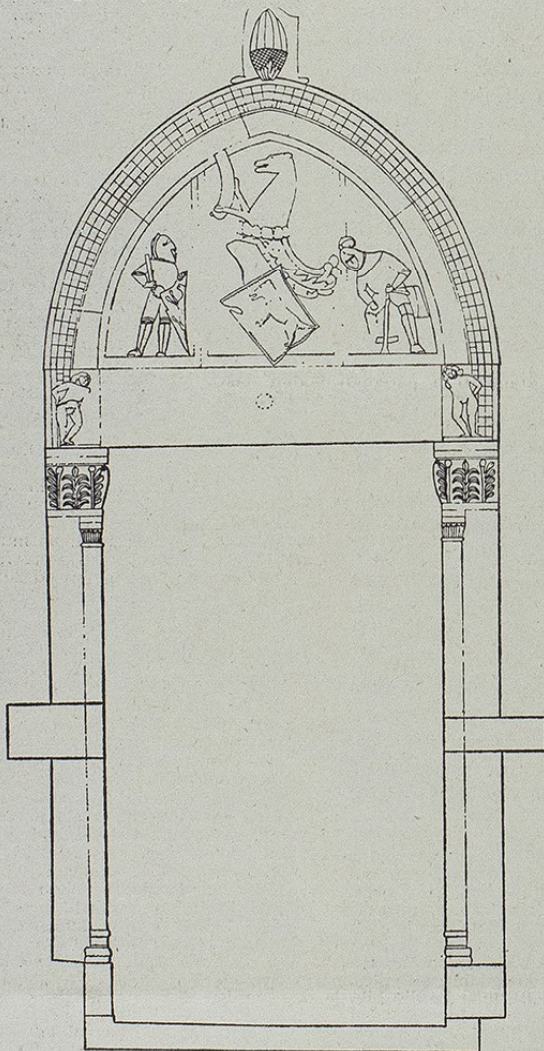
Gotički portal na kontaktu ulica J. Barakovića i 12. kolovoza 1941. Autor je fotogrametrijskog snimka inž. M. Kadi
